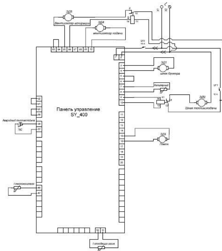
Электромонтажная схема.
